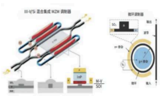
图：III-V/Si 混合集成 MZM 调制器和微环调制器结构
