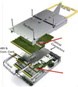
图：XPO核心架构拆解
